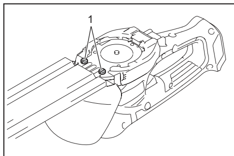
► 1. Screws
