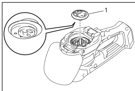
► 1. Crank
