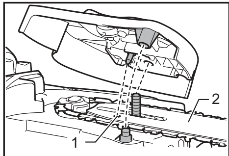
► 1. Hole 2. Guide bar
